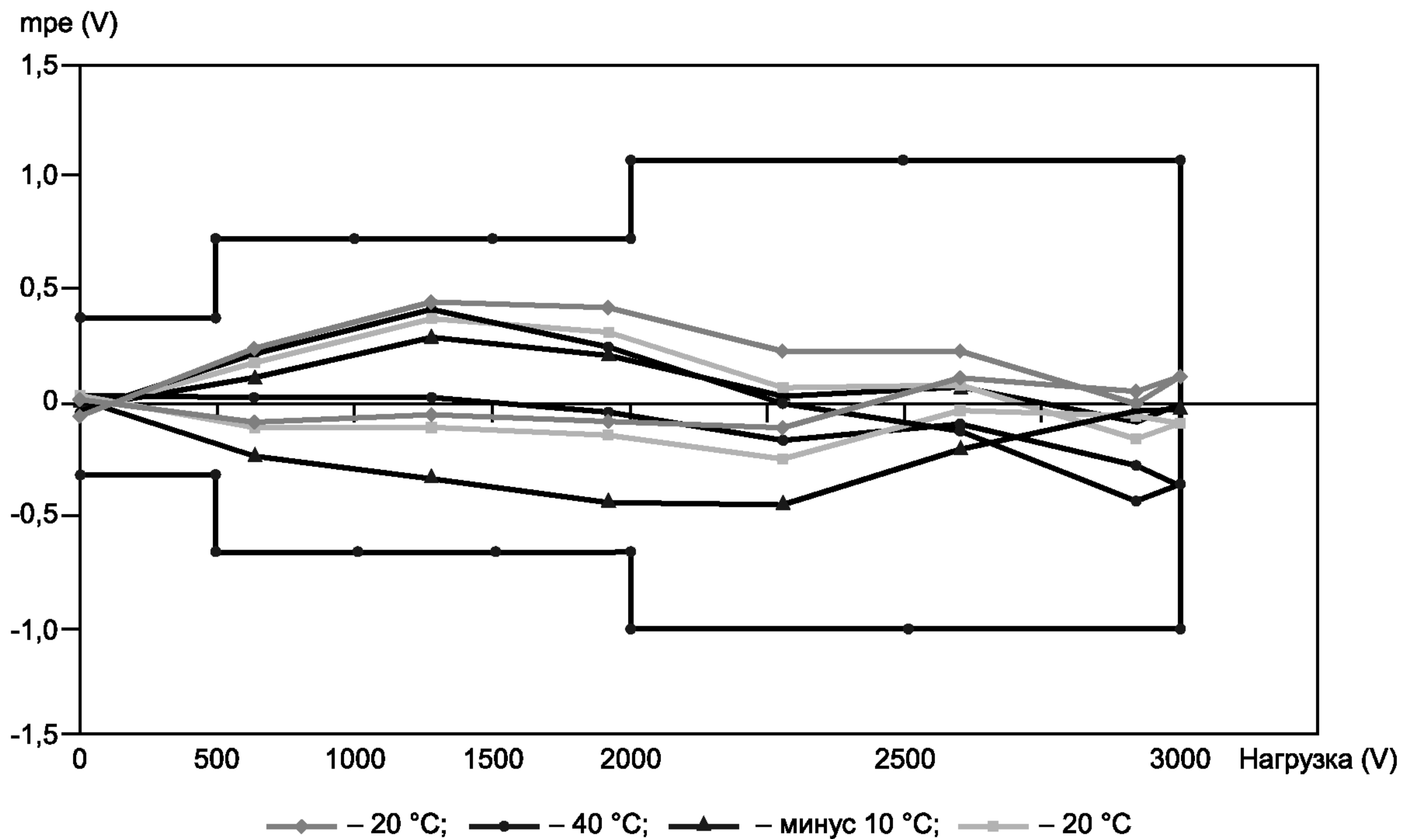
Рисунок С.1 — Пример кривой погрешности
